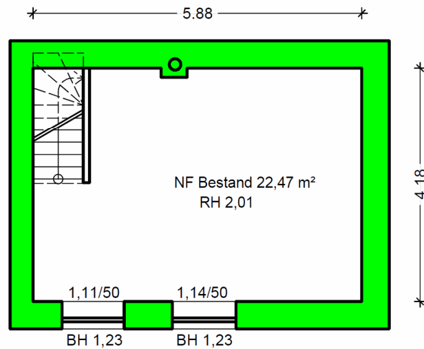
KELLERGEOSCHOSS BESTAND
