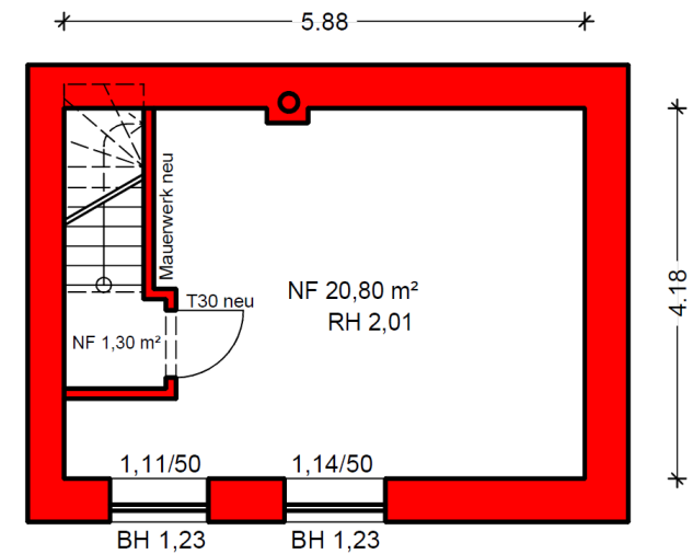
KELLERGEOSCHOSS PLANUNG
